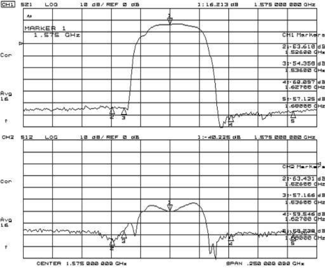
S21, S12
