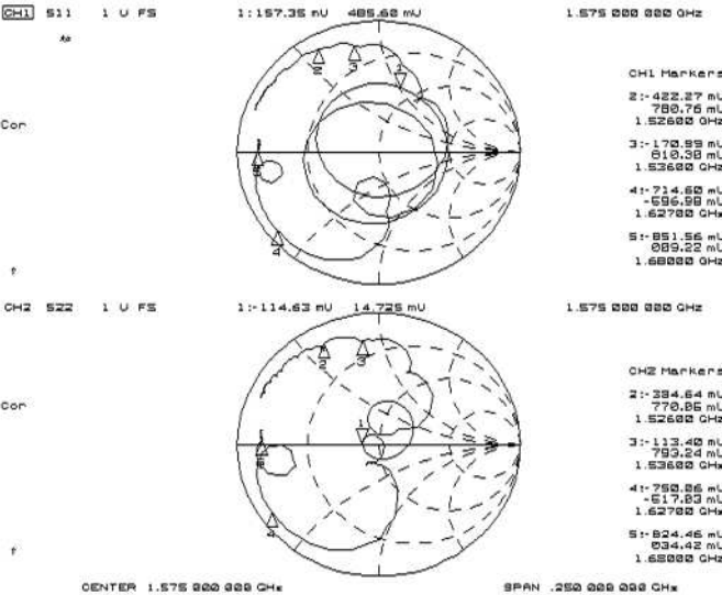
Zin, Zout
